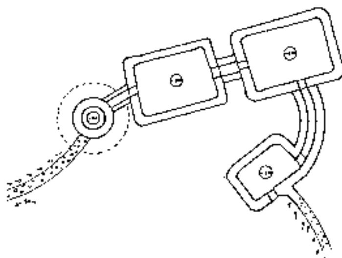
Fig. 4. Citerne à bassin: bouteille de décantation; deux bassins annexes décantation et stockage; deux bras d'alimentation (Oum el-Gueloub, Oued Kébir supérieur).
