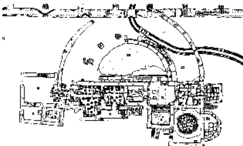
Fig. 8: S. Gielano di Vada (LI). Complesso termale. pianta.
