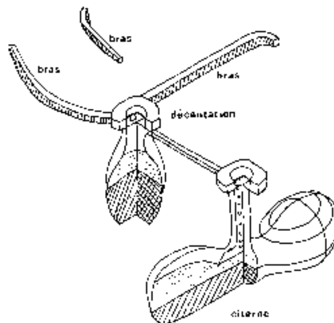
Fig. 6: Citerne «téléphone»: citerne à goullet et deux chambres; bouteille de dégorgation, avec canal de jonction; trois bras d'alimentation (Faschint en Nejeih, Oued Kehir supérieur).
