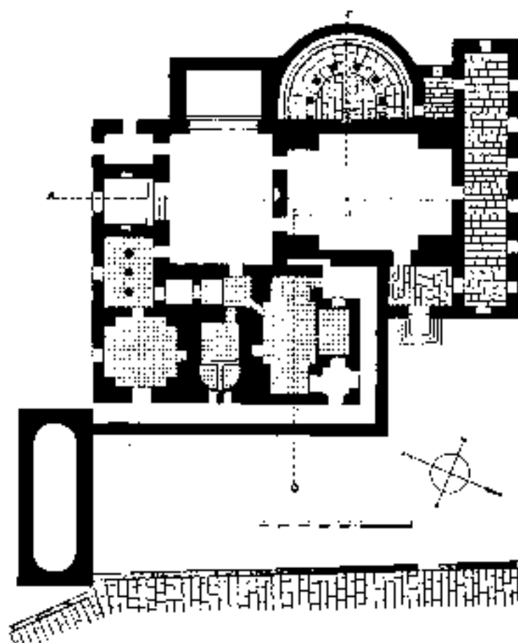
Fig. 4: Madauros (Algeria). Grandi Terme: pianta.
