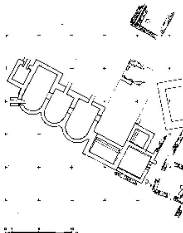
Fig. 7; Marrubiu (OR). Terme di «Muru de Bangius»: pianta.
