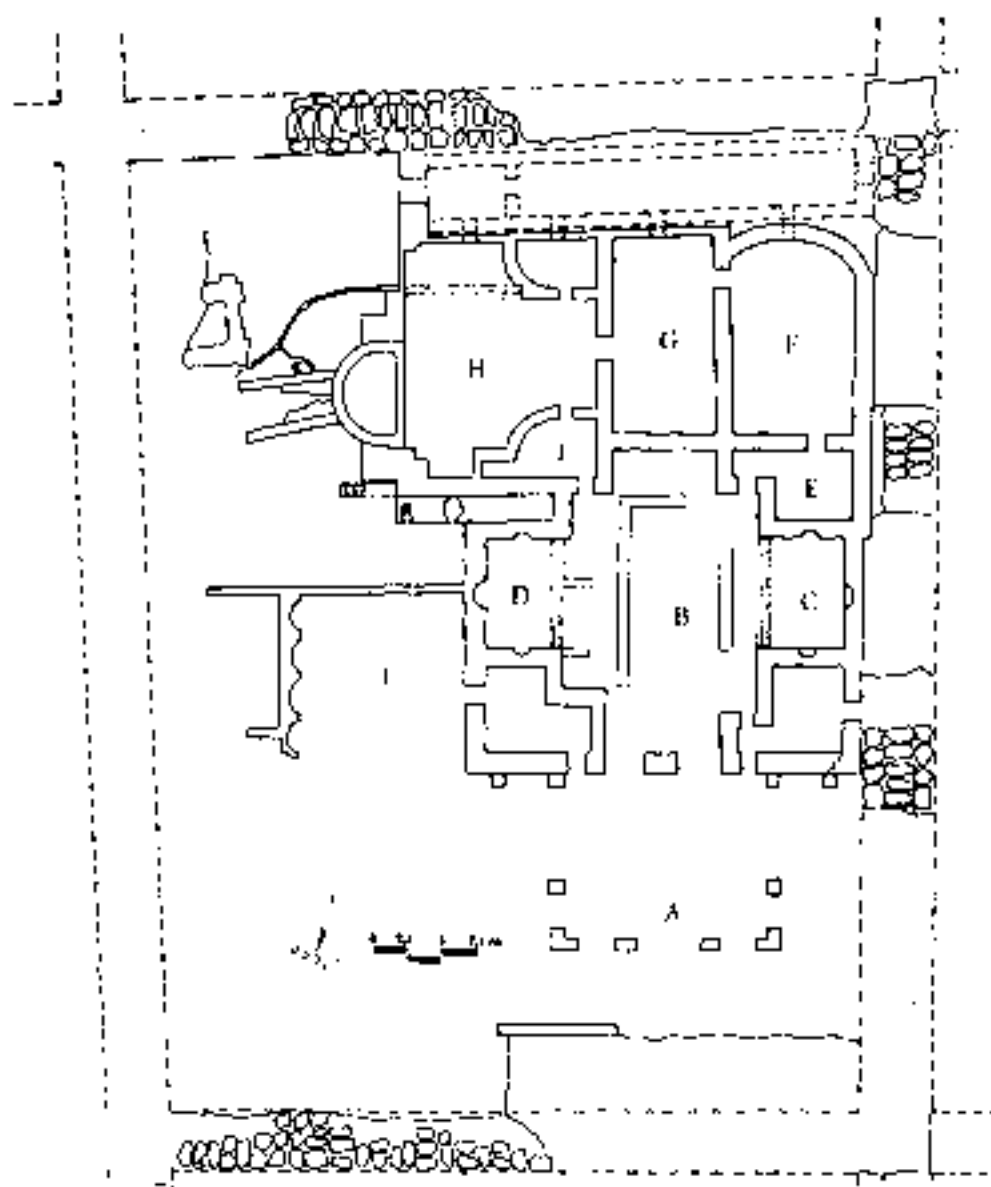
Fig. 5: Porto Torres (SS). Torre Centrale: pianta.
